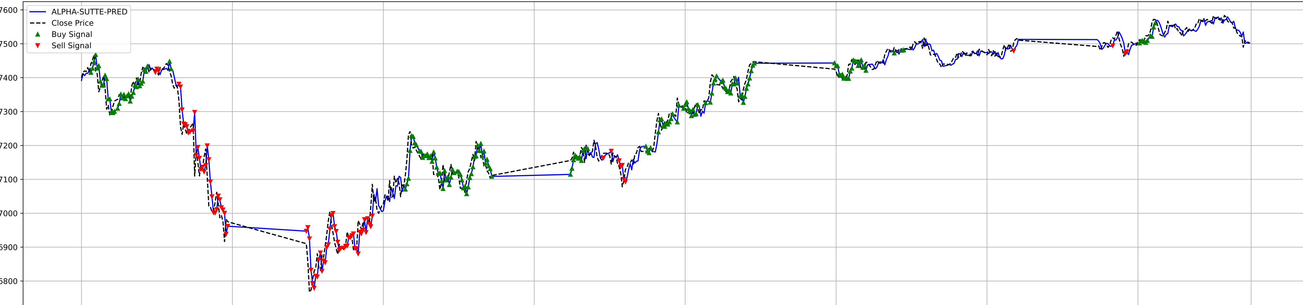
RSI
