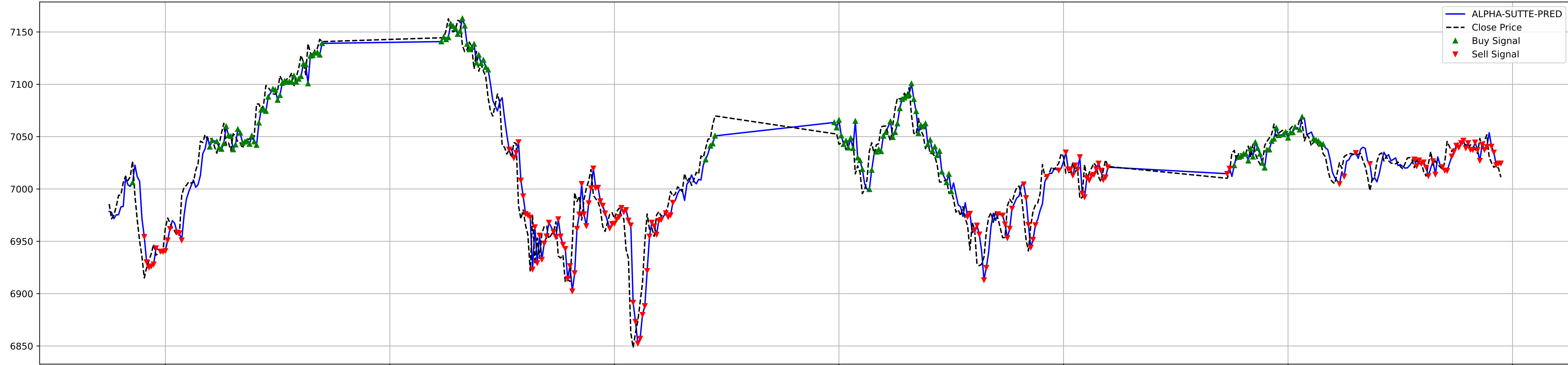
RSI
