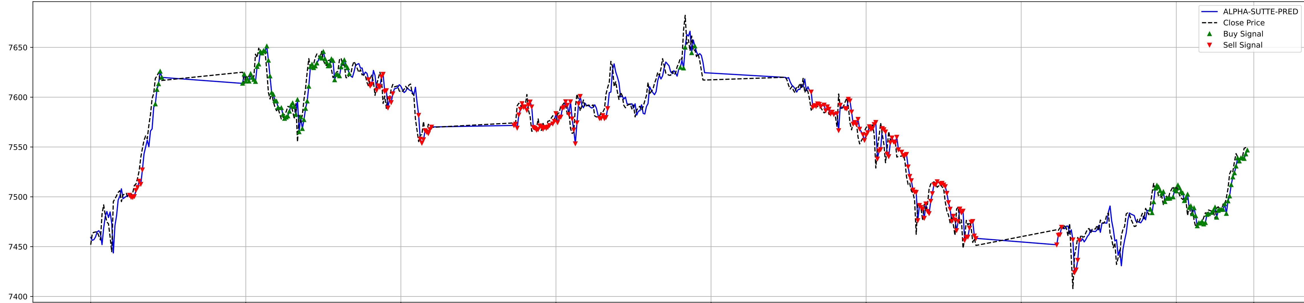
RSI
