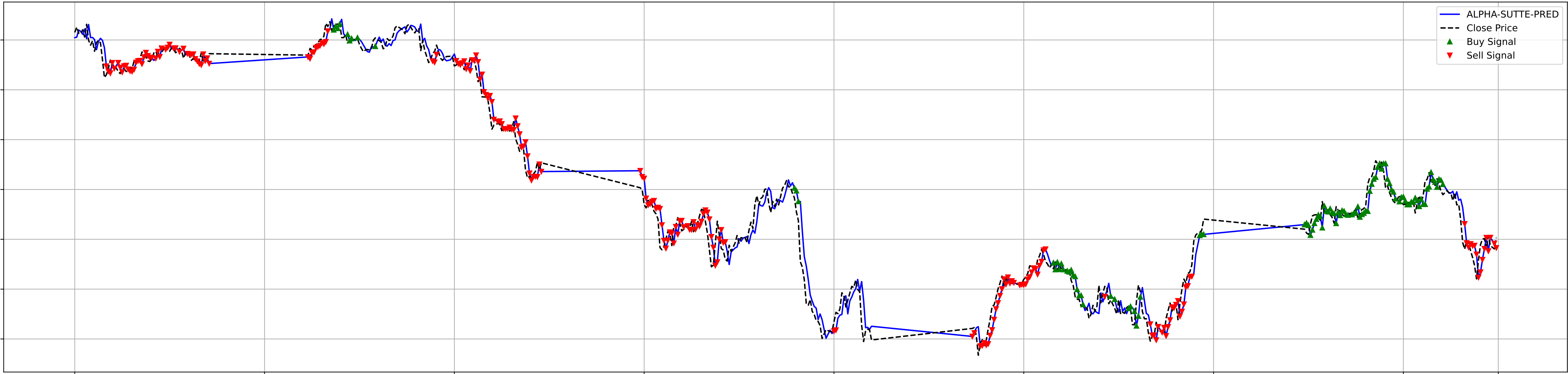
RSI
