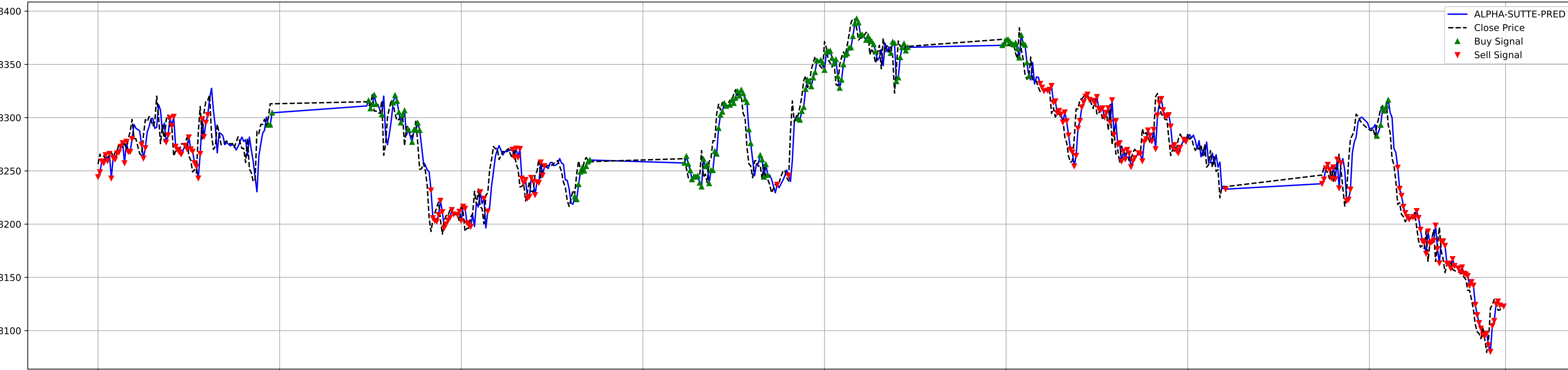
RSI
