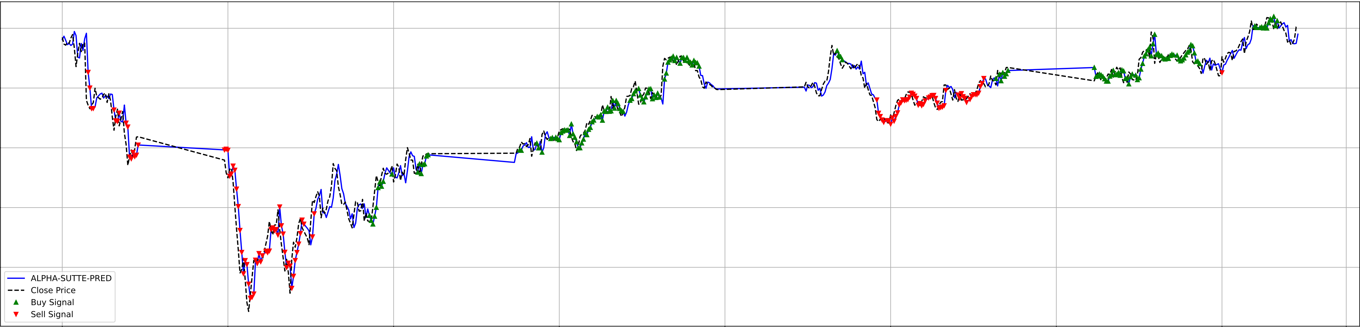
RSI
